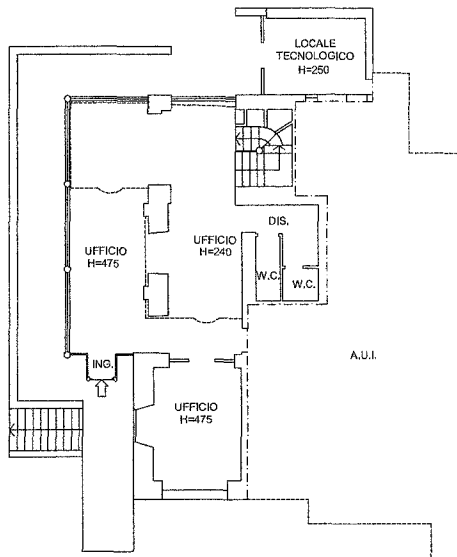
SECONDO LIVELLO SEMINTERRATO
